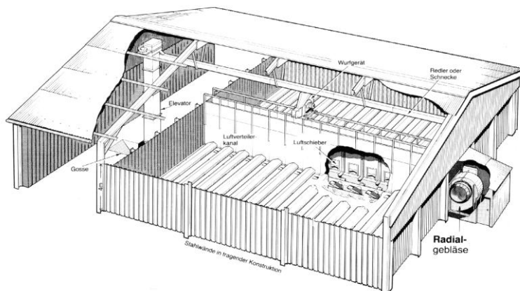
Getreideflachlager mit Belüftungstrocknung
