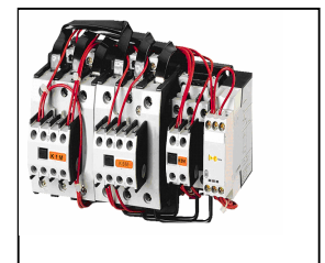
Schützschaltung Stern-Dreieck
